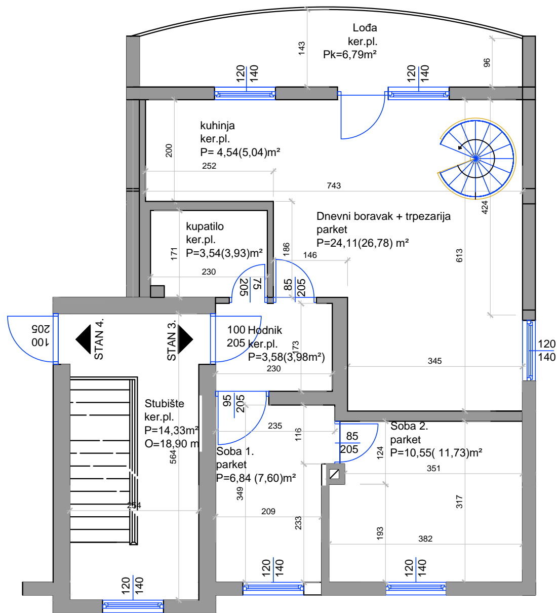
ETAŽA SPRAT, STAN 3.
