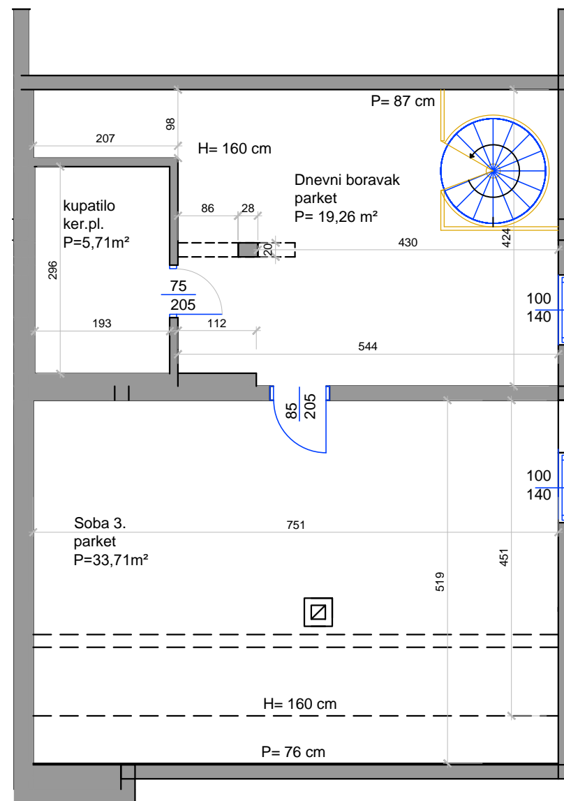
ETAŽA POTKROVLJE , STAN 3.
